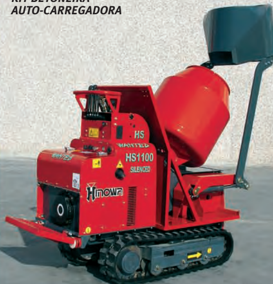
KIT HORMIGONERA AUTOCARGABLE KIT BETONEIRA AUTO-CARREGADORA
