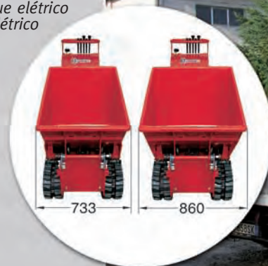
KIT CAJA AUTOCARGABLE CON DESCARGA ALTA KIT COM CAIXA DE CARGA AUTO-CARREGADORA DESCARGA ALTA
